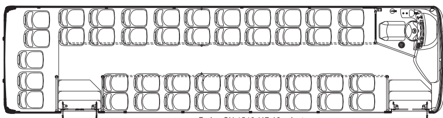
Torino OH 1519/47 43 asientos Torino OH 1519/52 47 asientos
