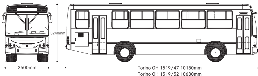
Torino OH 1519/47 43 asientos Torino OH 1519/52 47 asientos
